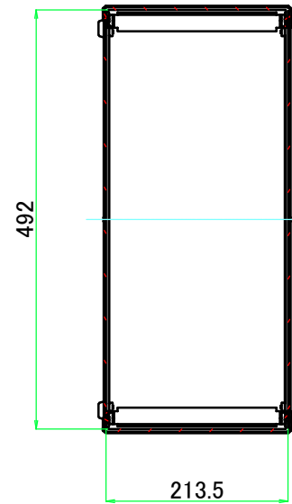
A-A ( 1 : 8 )
