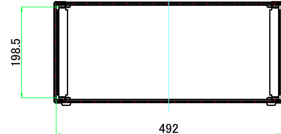
B-B ( 1 : 8 )
